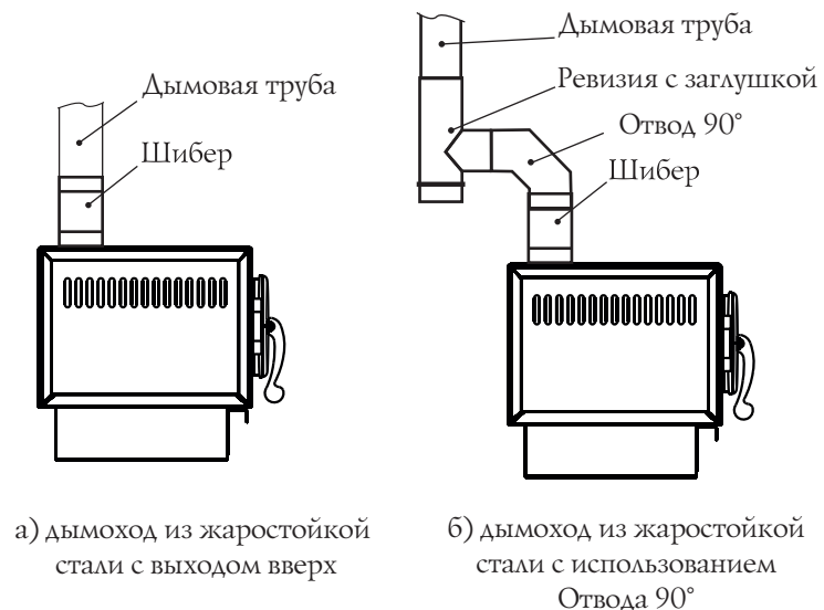
Рисунок 4. Схема присоединений печи к стальному дымоходу
